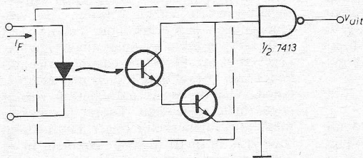
Fig. 2. Voorkomen van oscillaties bij langzame ingangsignalen door tussenschakeling van een schmitt-trigger.
