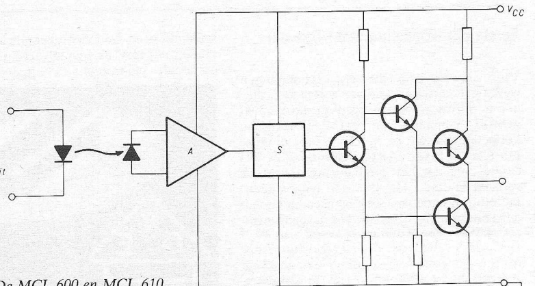
Fig. 59. De MCL 600 en MCL 610.
