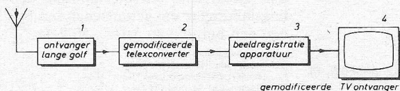
Fig. 24: Blokschema voor optisch-elektronische facsimile ontvangst.
