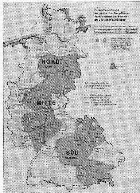
Fig. 1. Oproepbereiken EFuRD in West-Duitsland.
