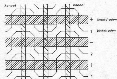
Fig. 3. Visualisering opbouw, met kanalen, houddraden en blokdraden.
