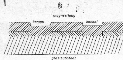
Fig. 1. Fysische opbouw van een DOT-geheugen.
