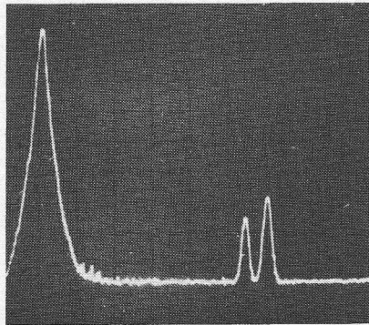
Afb. 1. Een groot frequentie bereik, samen met een hoog oplossend vermogen, stellen de gebruiker in staat om dicht op elkaar staande spectrum lijnen van elkaar te onderscheiden. Op de afb. een 10 kHz signaal met 60 Hz (netspanning) en 54 Hz (veroorzaakt door een ventilator) zijbanden. Vert.: 10 dB/div., hor. 10 Hz/div.
