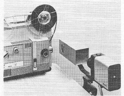
Afb. 11. Philips telecine adapter met standaardcamera LDH 25.
