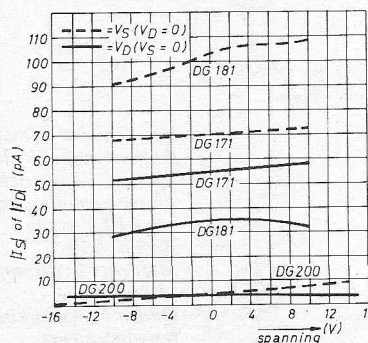
Fig. 4. Foutstromen in enkele FET-schakelaars.
