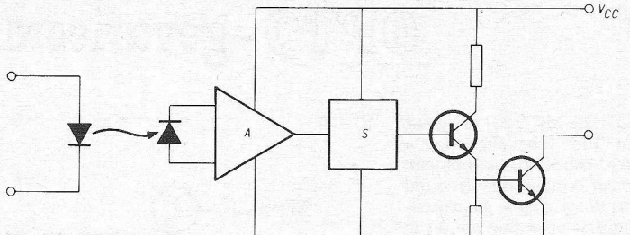
Fig. 5b. De MCL 601 en MCL 611.
