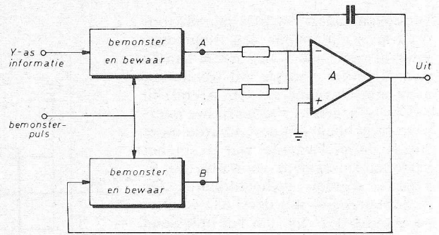
Fig. 8. De uitgangsspanning van de integrator is evenredig met het verschil van twee opeenvolgende Y-waarden.
