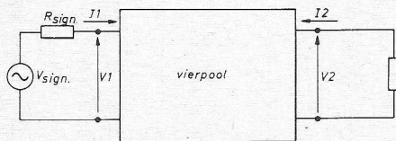
Fig. 3. Gelijkspannings-vervangingschakelingen. Vbvb.: Algemeen, voor de uit- en voor de aan-toestand.
