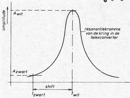
Fig. 27. Omzetting van frequentievariatis in amplitudevariatis (Flankdemodulatie).
