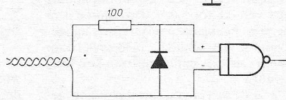
Fig. 8. Lijnontvanger.
