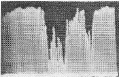
Afb. 25. Oscilloscoopbeeld van het enkelfasig gelijkgerichte facsimile signaal bij negatieve beeldvorming.
