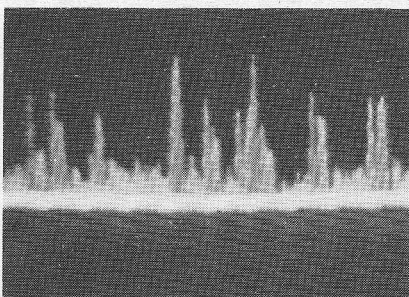
Afb. 23. Oscilloscoopbeeld van het enkelefasige gelijkgerichte facsimile signaal bij positieve beeldvorming. Maximale amplitude komt overeen met wit en minimale amplitude met zwart. Door het weg laten van het RC-filter worden de snelle amplitude variaties niet afgevlakt; dit doet de beeldscherpte toenemen.
