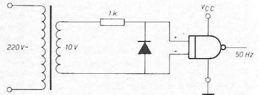
Fig. 9. Signaalbegrenzer.
