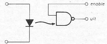
Fig. 10. Schemasymbool van de 5082-4360.
