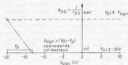
Fig. 7. Aan-schakeltoestand.
