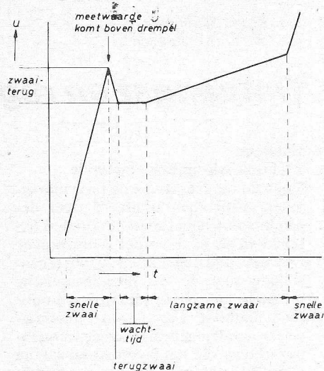
Fig. 11. Tijdfunctie van de veranderlijke zwaai. De grootte van de terugzwaai is afhankelijk van de bandbreedte - en zwaaitijdinstellingen.
