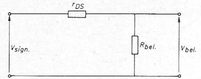
Fig. 6. Fout door schakelaar-AAN weerstand.
