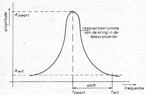
Fig. 29. Afstemming van de beatoscillator bij negatieve beeldvorming.
